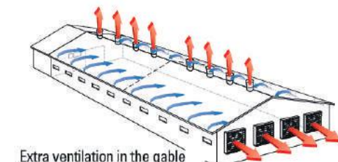
Longitudinal ventilation
