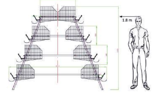
160 CAGE
